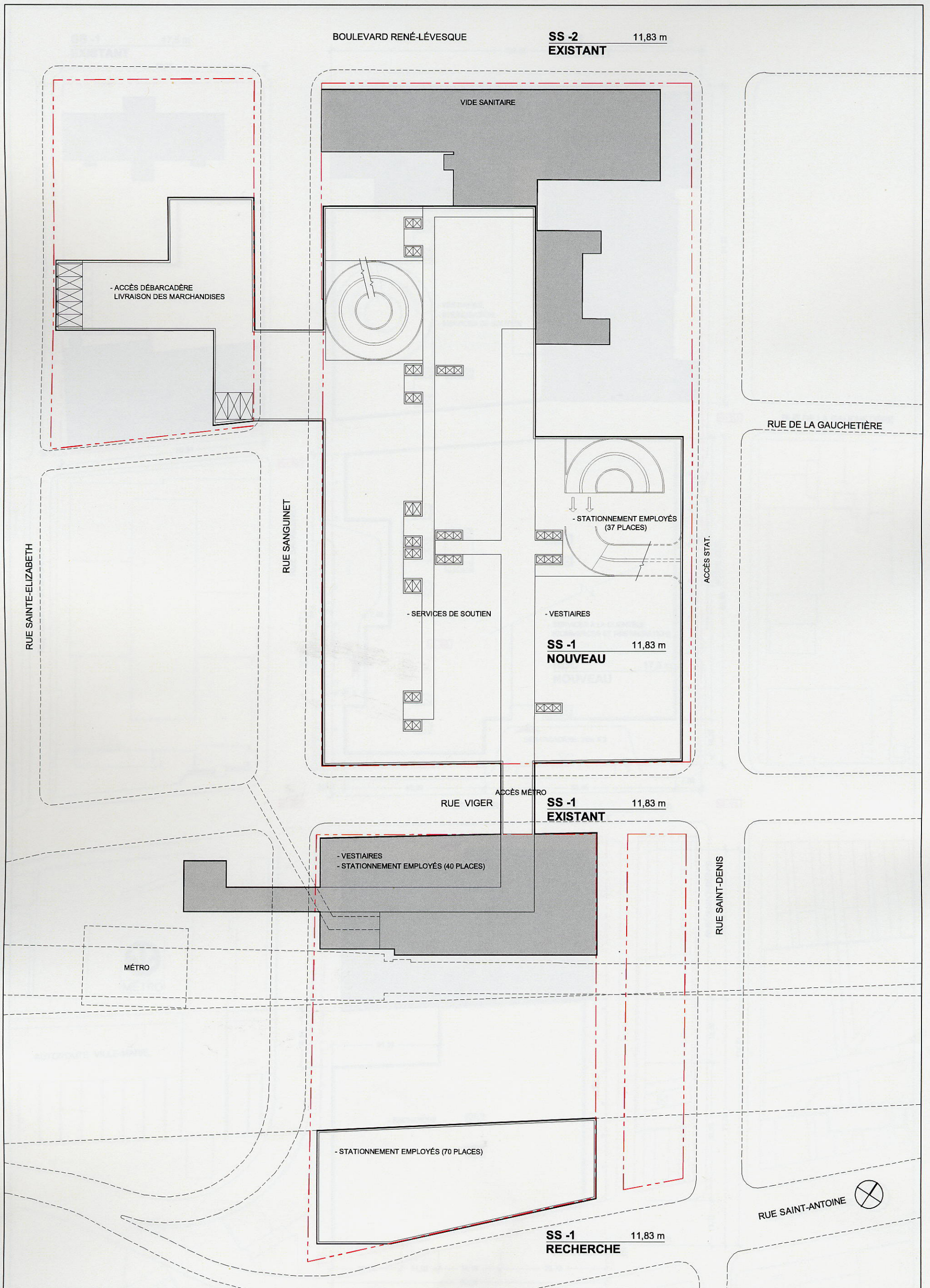
Plan projeté niveau SS-1 Nouveau pavillon
