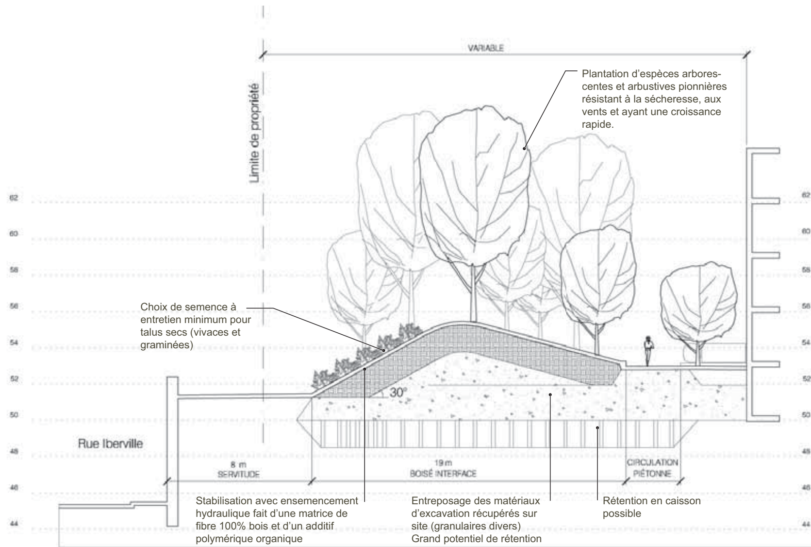
Coupe technique
